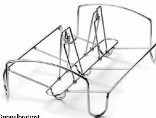
Doppelbratrost Art.-Nr. 74 6791 Maß 12 x 34.5 x 26 cm Material Edelstahl EAN 0065506067919 VE 4
